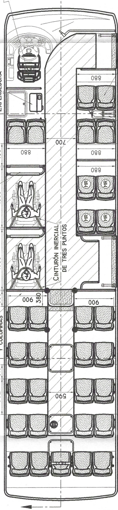
ALTERNATIVA B 29-31 ASIENTOS
