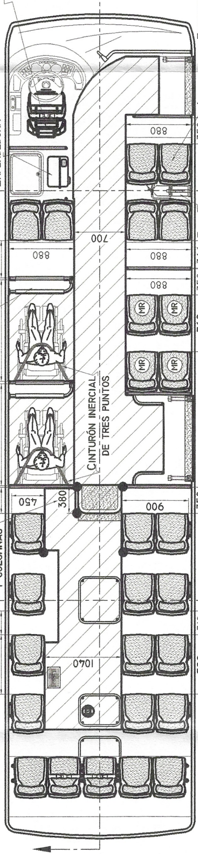
ALTERNATIVA A 25-27 ASIENTOS
