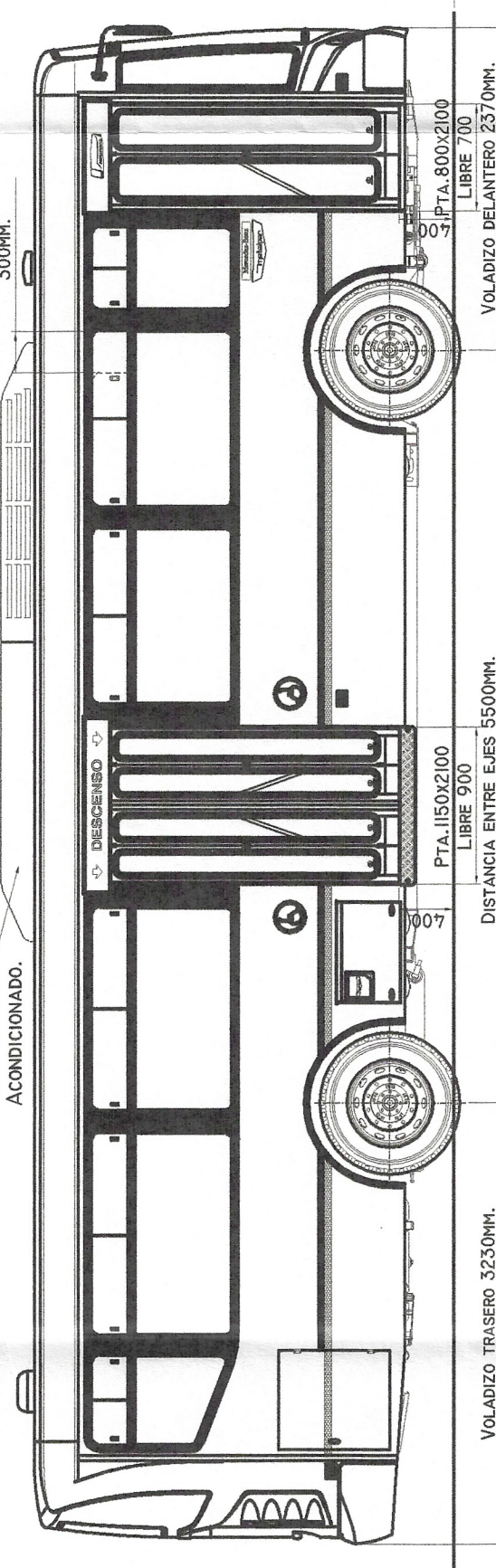
VISTA LATERAL DERECHO
