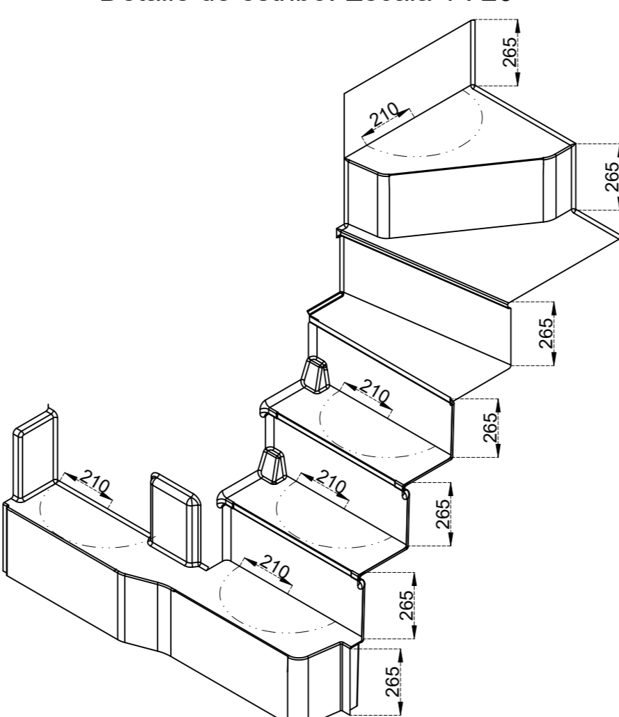
Detalle de estribo: Escala 1 : 20
