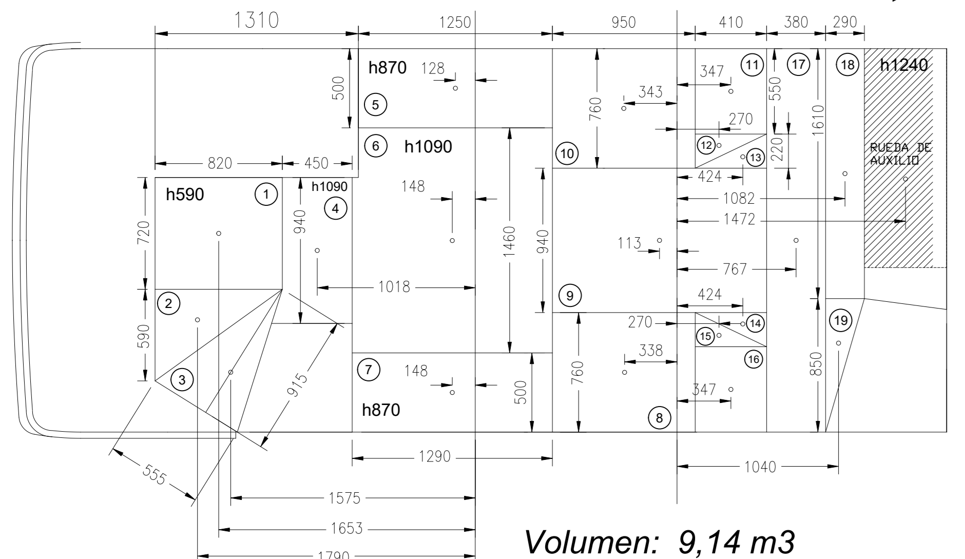
Detalle de Portapaquete: Escala 1 : 10
