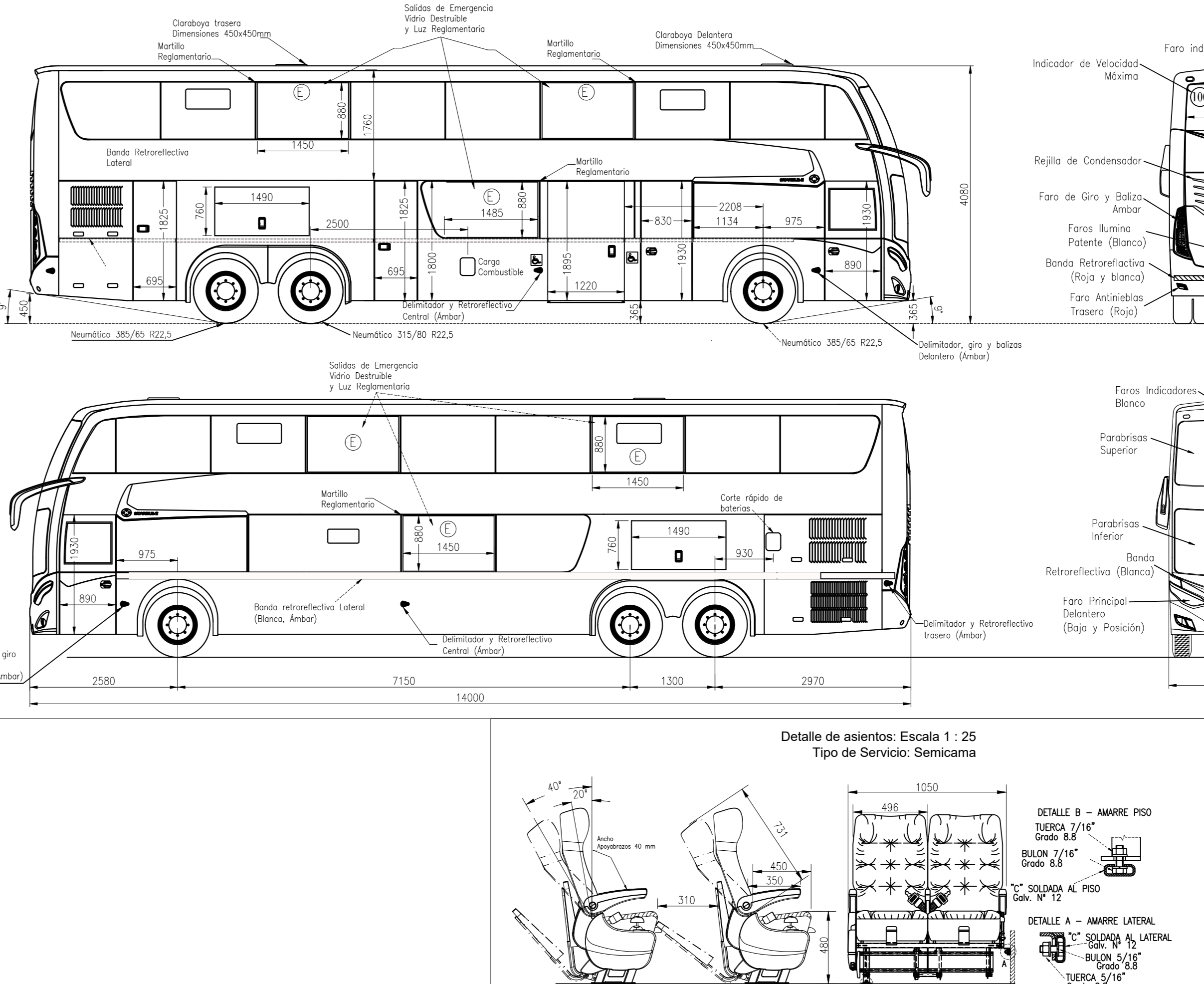
PISO INFERIOR: 11 Asientos SEMICAMA + Conductor + Acompañante + Baño
