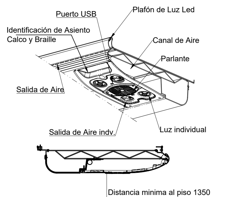
Detalle de Portapaquete: Escala 1 : 10
