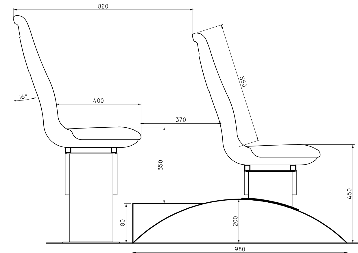
DETALLE ASIENTOS SOBRE PASARRUEDAS TRASERO IZQUIERDO (Esc.: 1:10)
