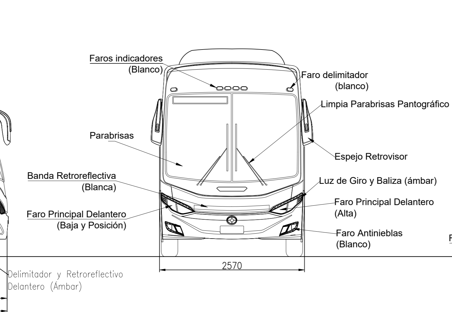
Vista Frontal Escala 1 : 50
