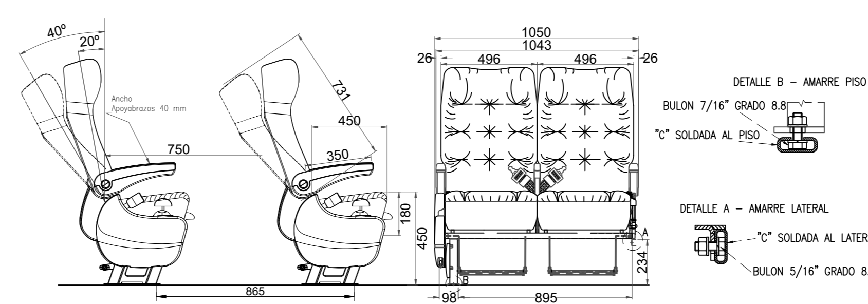
Detalle de asientos: Escala 1:10 Tipo de Servicio: Común
