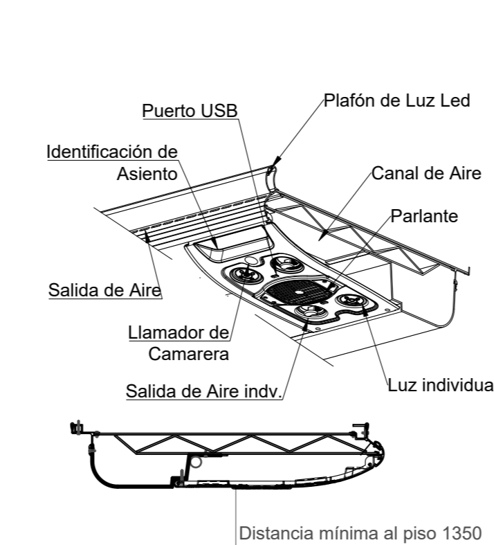
Detalle de Portapaquete: Escala 1 : 10
