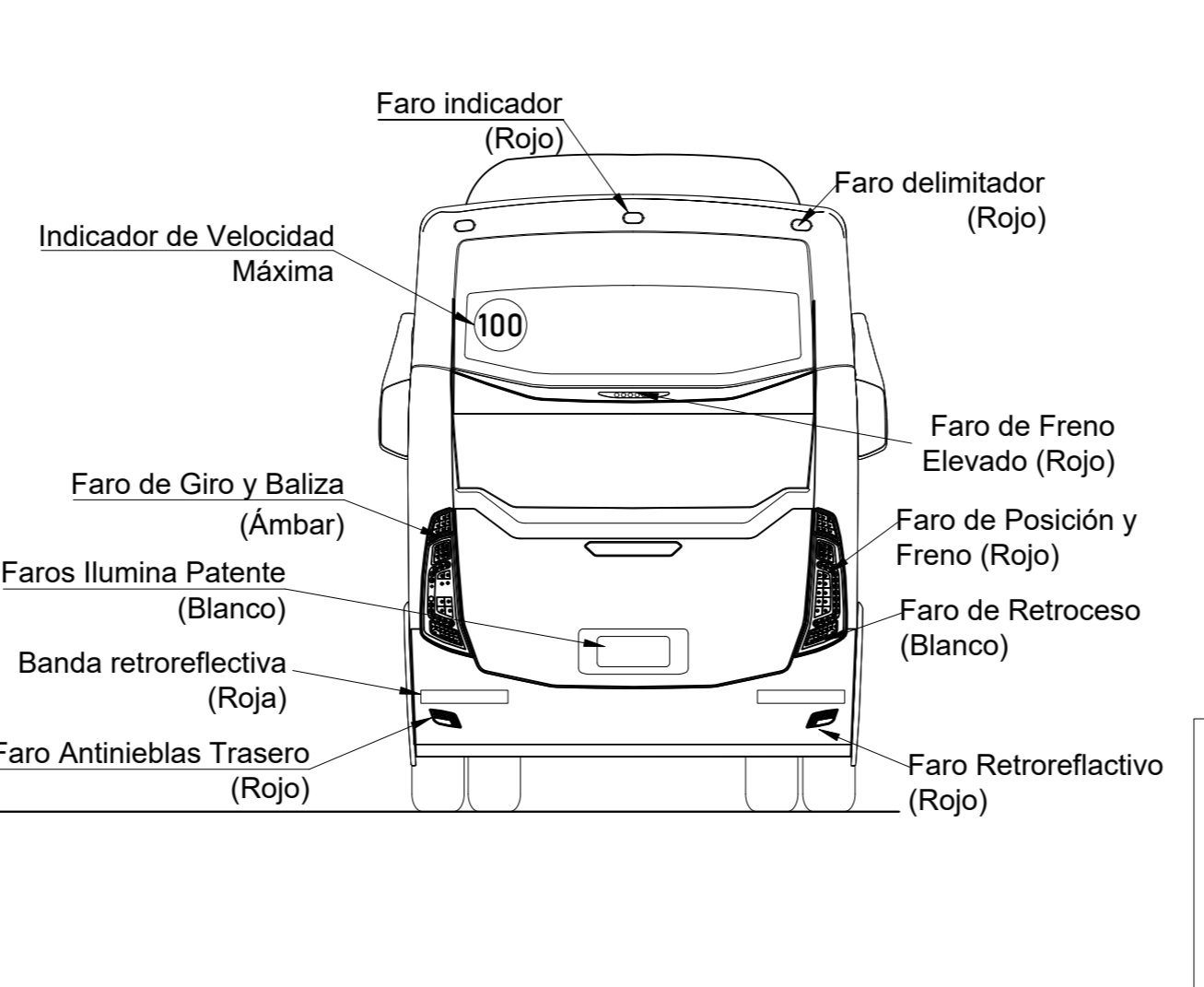
Vista Posterior Escala 1 : 50
