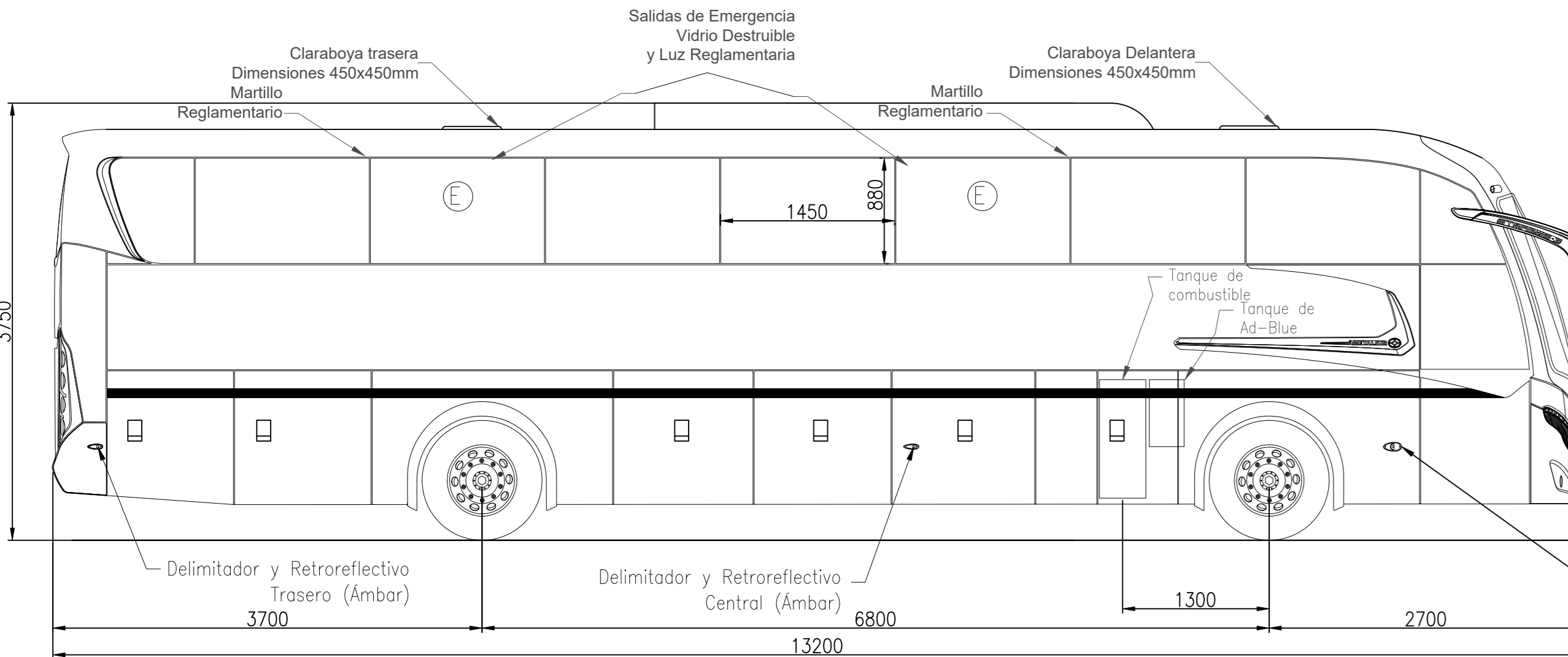
Vista Lateral Escala 1 : 50
