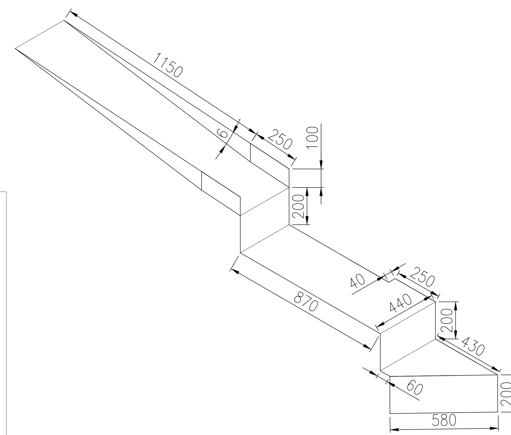
Detalle de estribo 2 Escala 1:10
