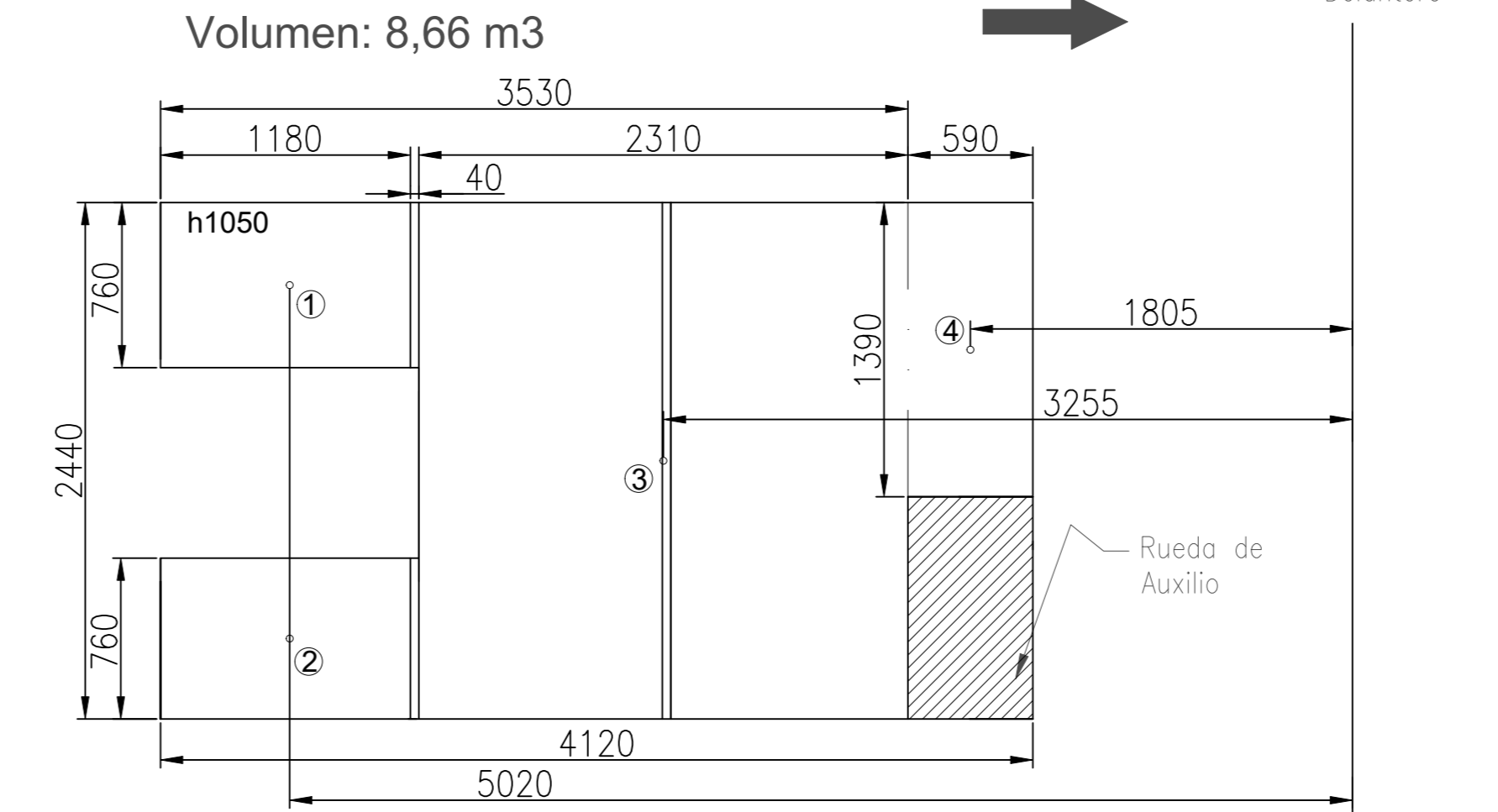
Detalle de bodega Escala 1:30 Volumen: 8,66 m3
